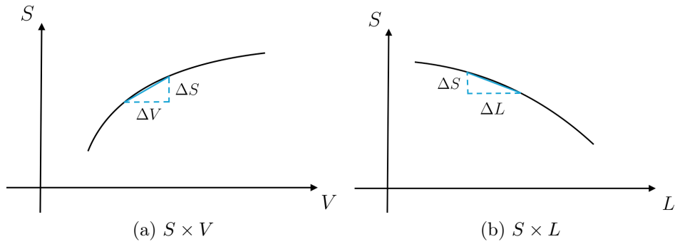
Figura 5.4: (a) Entropia em função do volume para um gás ideal. (b) Entropia em função do comprimento para uma borracha ideal.
